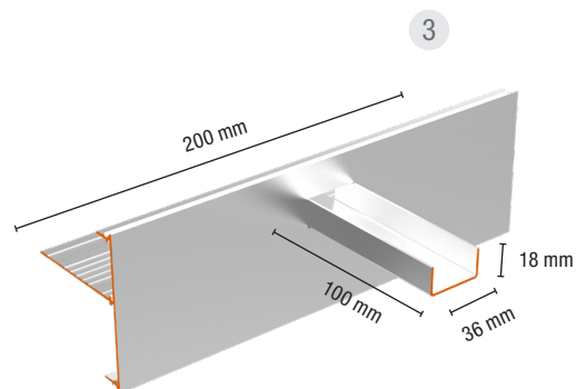
standaardspuwer
