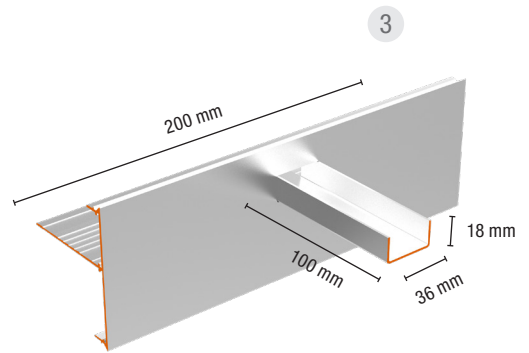
gargouille standard
